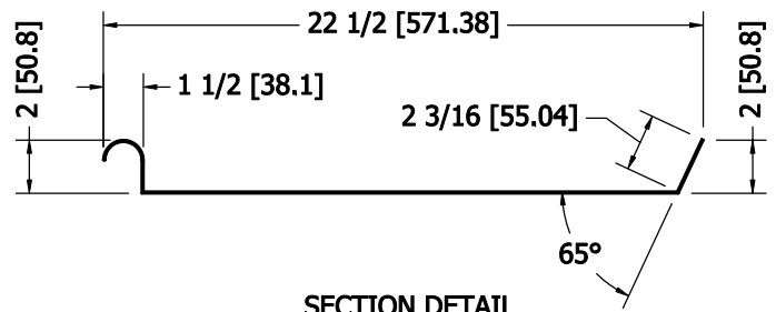
SECTION DETAIL Scale: N.T.S.
